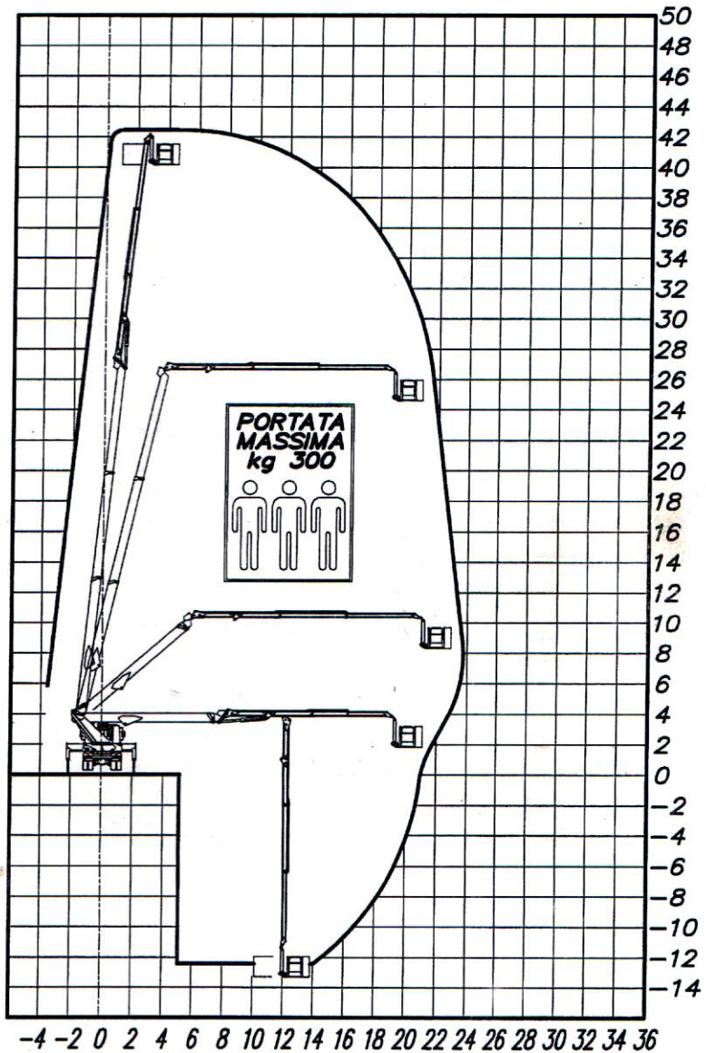
SIoux TJ 42 Installazione su veicolo PTT 26t Stabilizzazione ridotta
